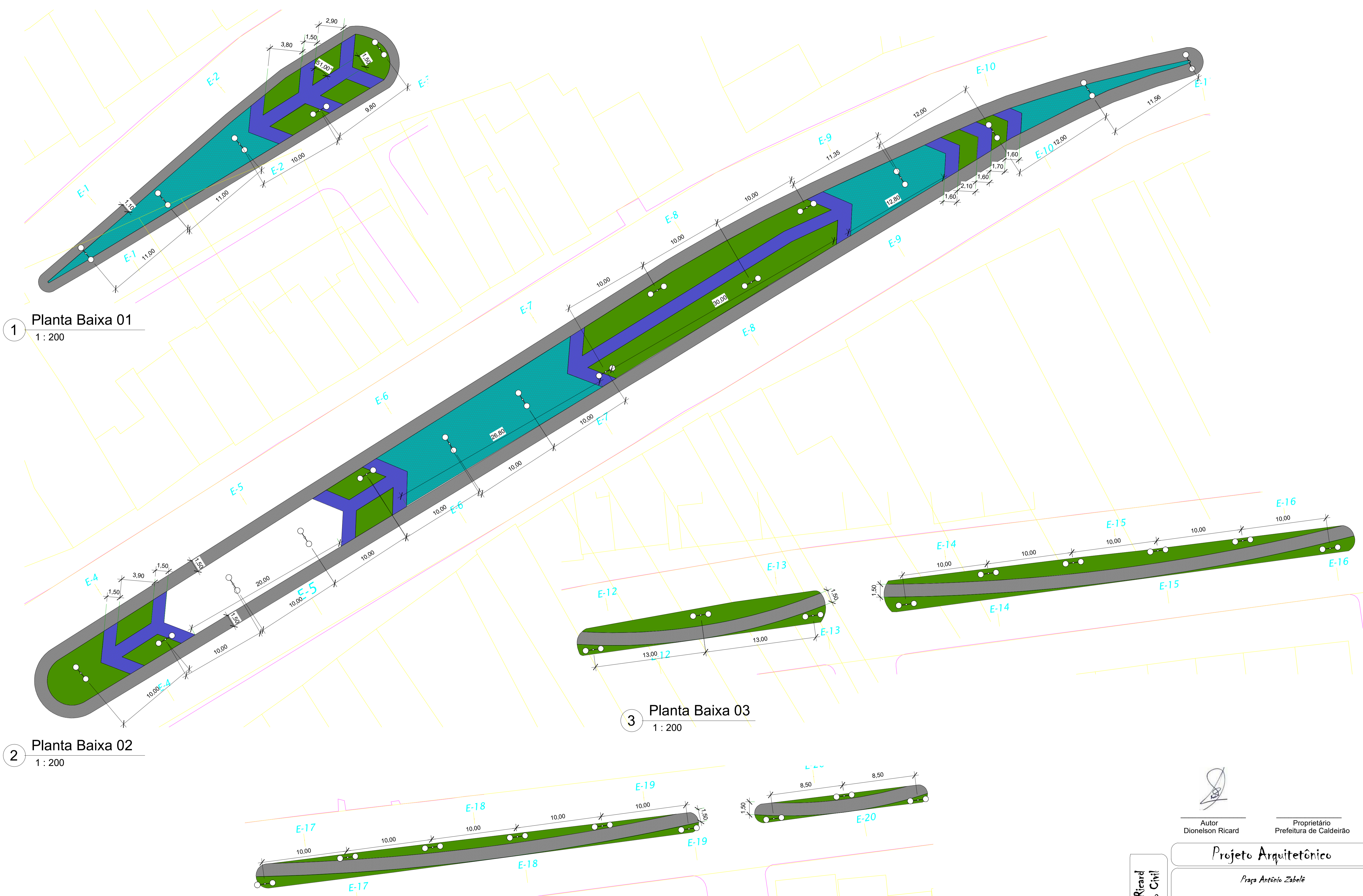
4 Planta Baixa 04 1 : 200
